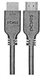
CABO HDMI 2.0 4K 28AWG PURO COBRE 5 METROS - PHM20-5
